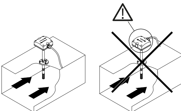
Fig. 2 La direzione della freccia deve coincidere con quella del flusso.
