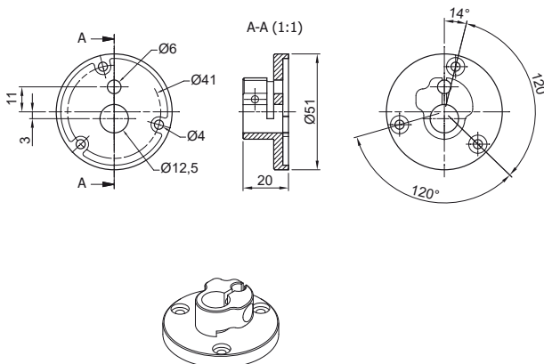
Fig. 4 Dimensioni della staffa di montaggio
