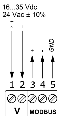
Fig. 6 Cablaggio elettrico per Modbus rtu
