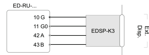
Figur 2 Inkoppling med en EDSP-K3-kabel
