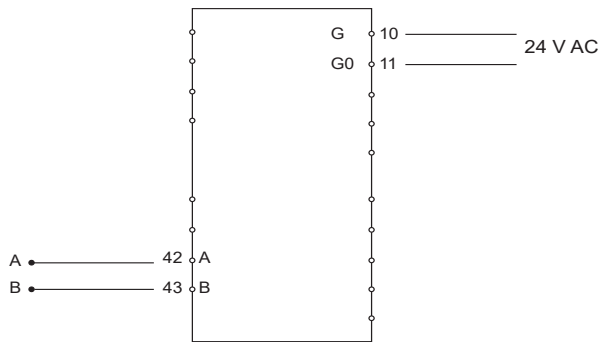
Bild 1 Verdrahtung
